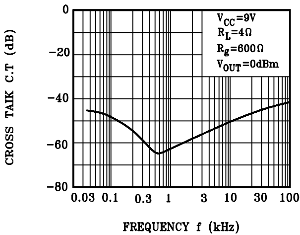
C.T - f
